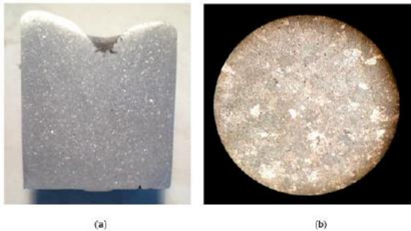
Fig.11. – Al-3% Cu - Corte transversal, 20X.
