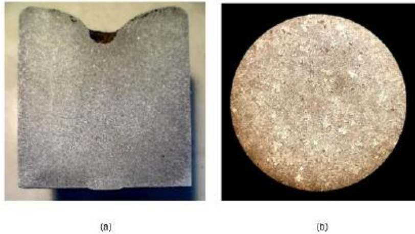
Fig.12. –Al-5% Cu - Corte transversal, 20X.
